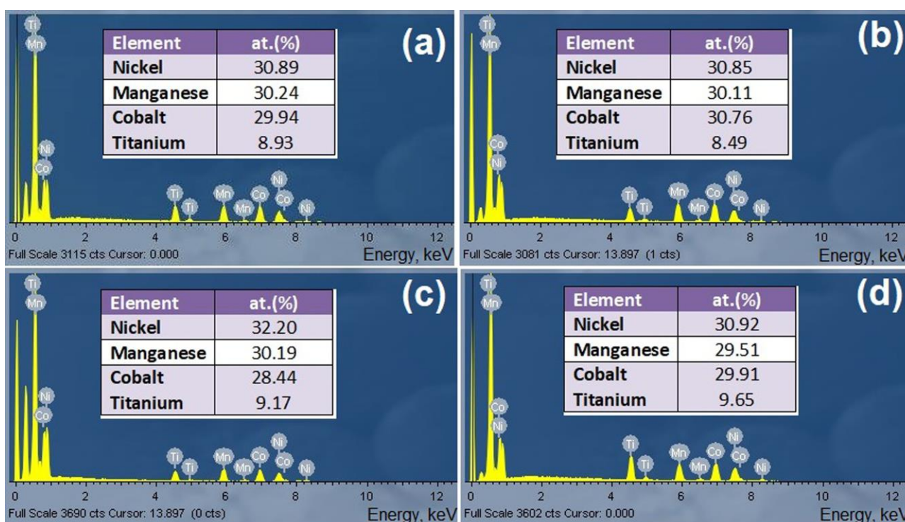
Figure S-1. EDX spectra of (a) T65 (b) T70 (c) T75 and (d) T80
